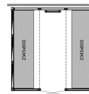
PANACEA 2525 2B Abmessungen: 2525 x 2525 x 2090 mm
