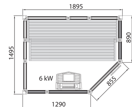
IMPRESSION-SAUNAKABINE I1915/C
