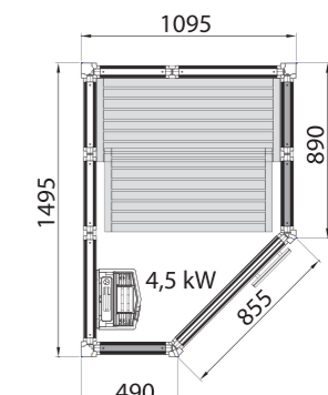
IMPRESSION-SAUNAKABINE I1115/C
